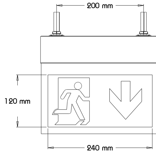
Ansicht Hinten
